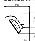
Vue latérale (avec déflecteur de chaleur)
