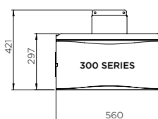
Vue de face (sans déflecteur de chaleur)
