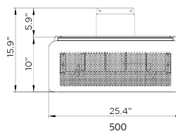
VUE AVANT (SANS DÉFLECTEUR DE CHALEUR)
