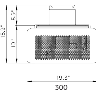
VUE AVANT (SANS DÉFLECTEUR DE CHALEUR)
