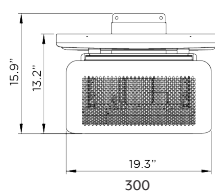
VUE AVANT (AVEC DÉFLECTEUR DE CHALEUR)
