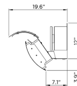
VUE LATÉRALE (AVEC DÉFLECTEUR DE CHALEUR)
